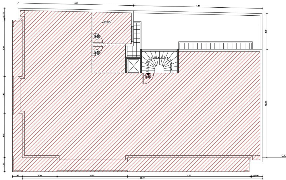
Σχέδιο 1. Κάτοψη δώματος στο οποίο θα πραγματοποιηθούν εργασίες.
